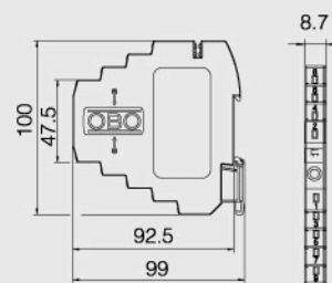
MDP尺寸图
