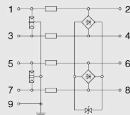
MDP结构图
